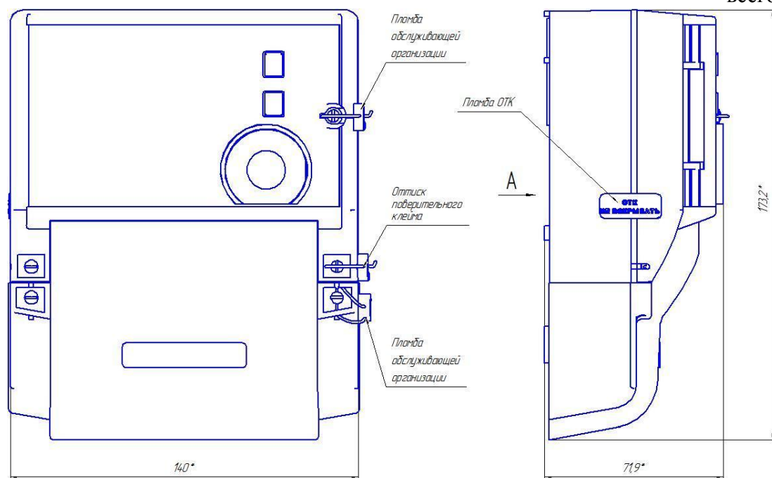
Рисунок 2 – Схема пломбирования счётчика
